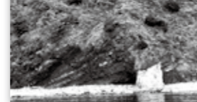
溶岩流でできた岩盤(鮎島湾・大岡)
