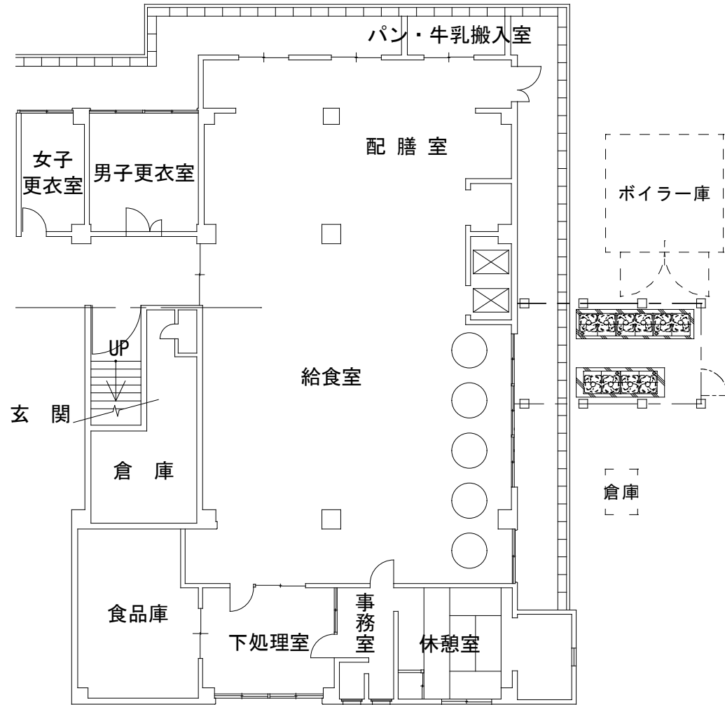
【沼津市立今沢中学校共同調理場 平面図】
