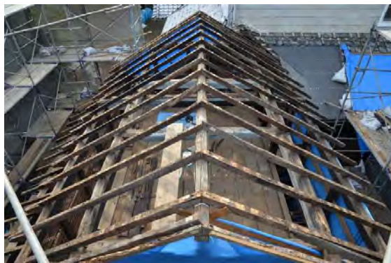
ミ解17 大屋根垂木状況
