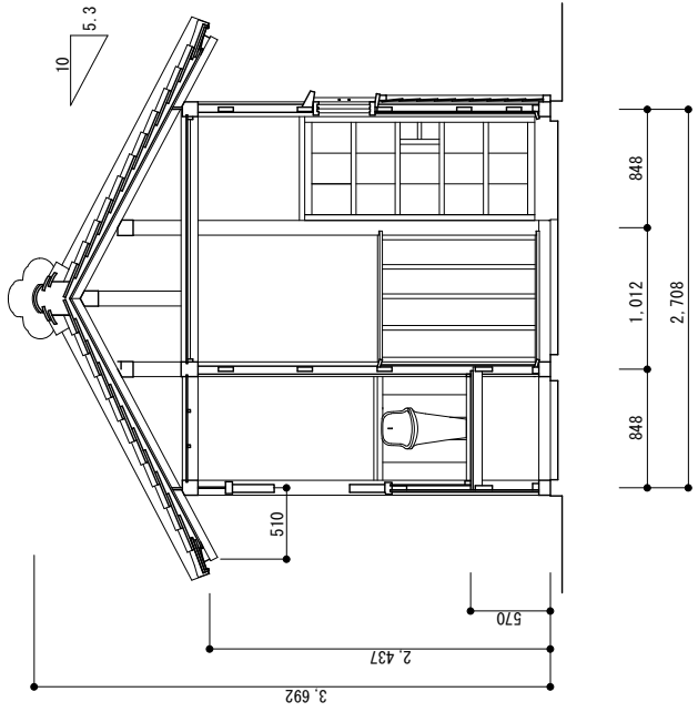
梁間断面図
