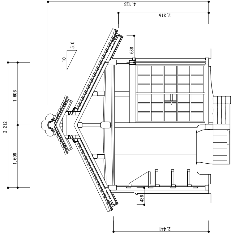
梁間断面図
