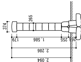
庭塼 断面図
