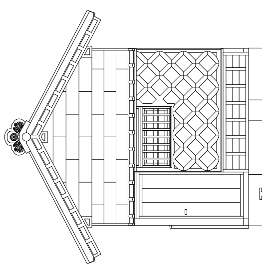
西立面图
