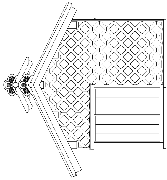
東立面図
