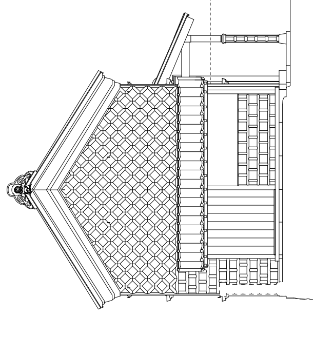
北立面図
