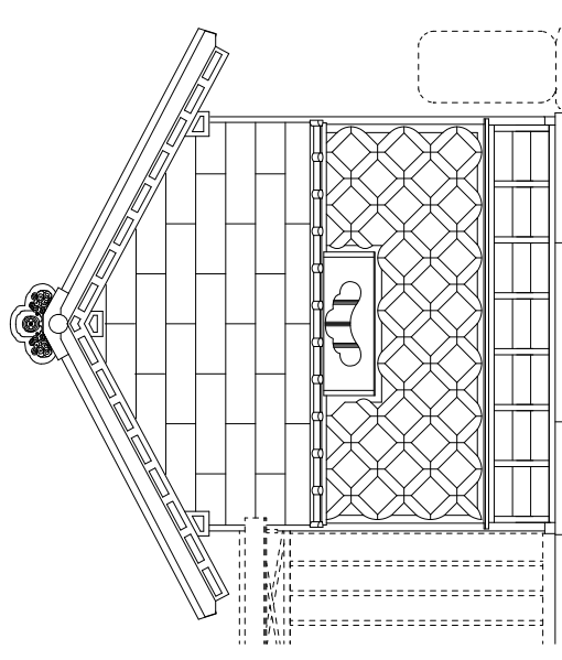
西立面图
