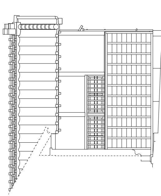
北立面图
