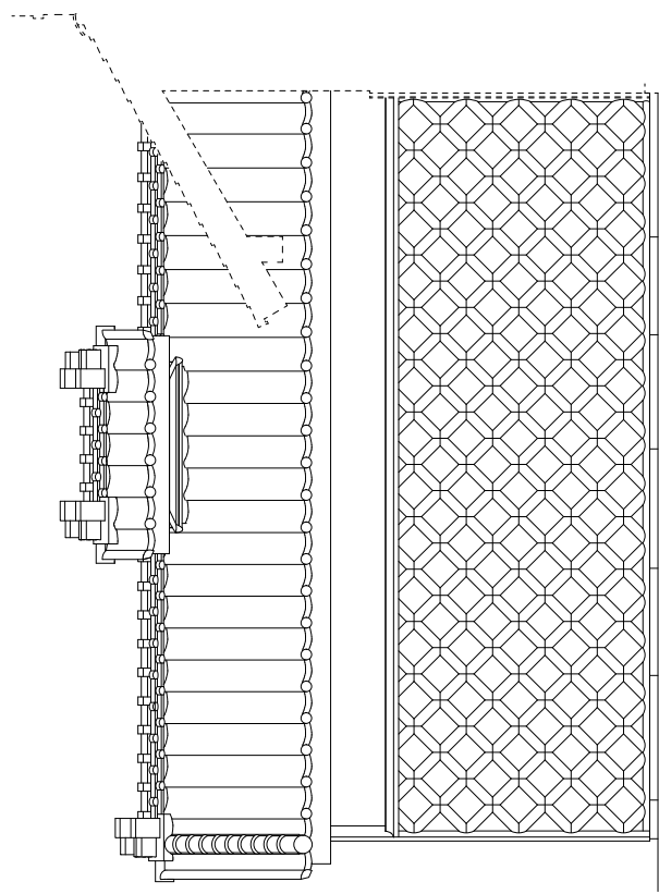
南立面図
