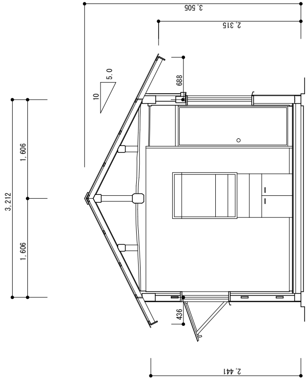
梁間断面図
