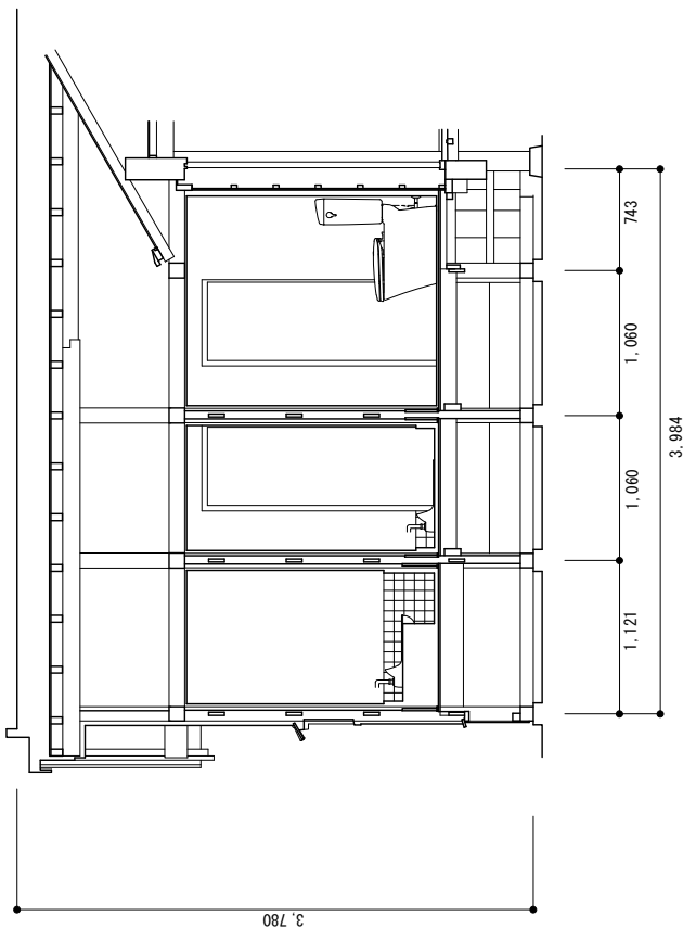
桁行断面図
