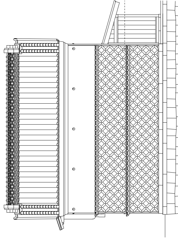
西立面図
