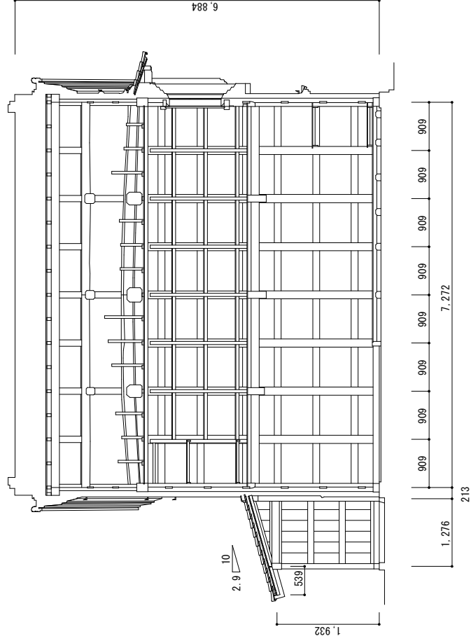
桁行断面図
