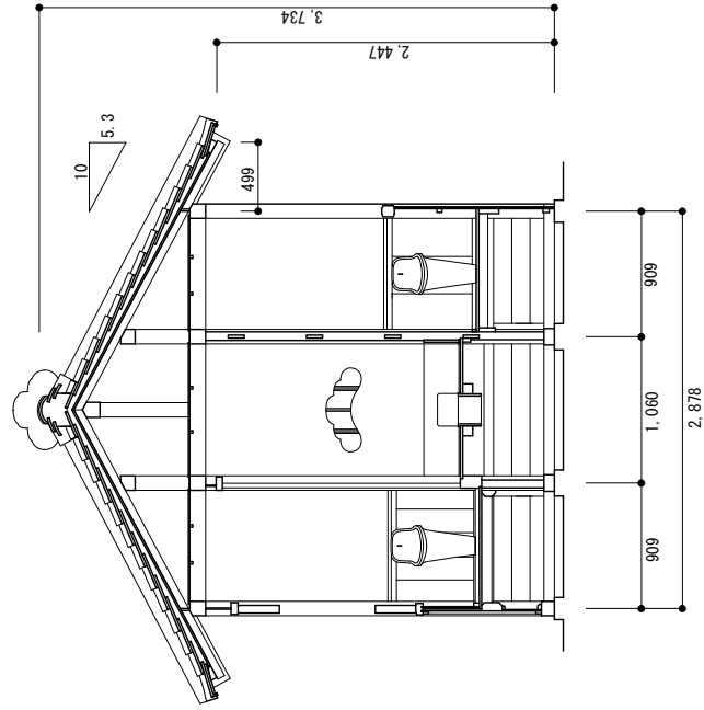
梁間断面図
