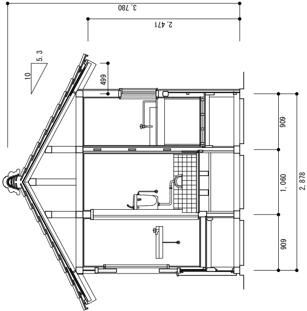
梁間断面図
