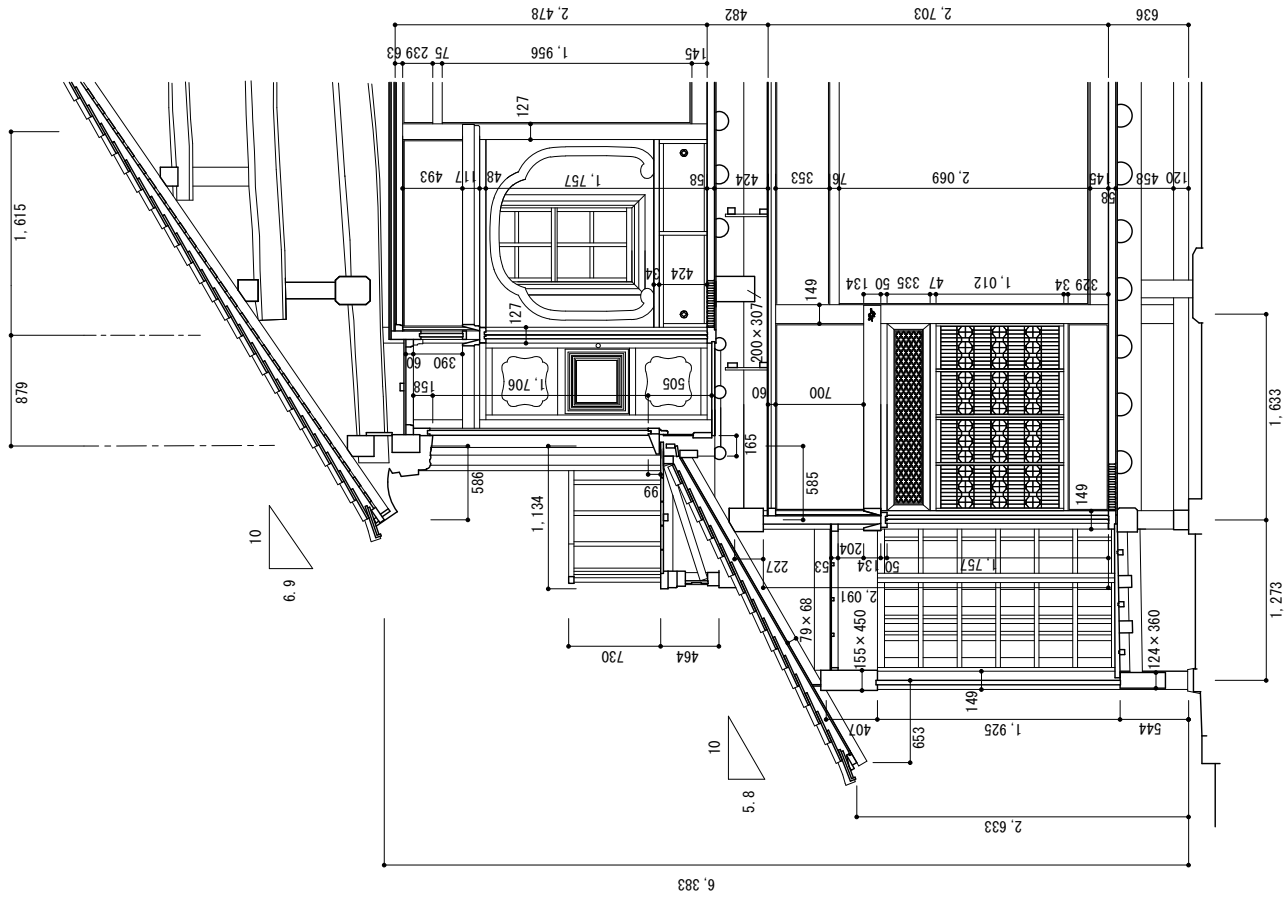
梁間南側矩計図
