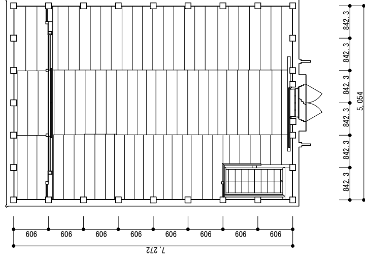
二階平面図
