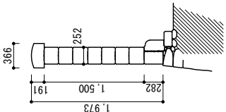
北塼 断面図
