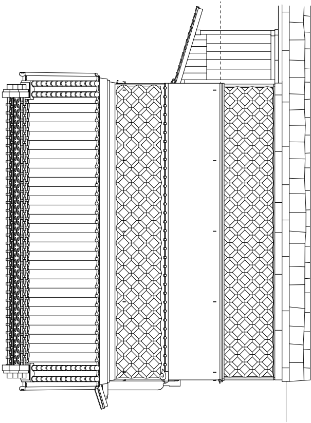
西立面図
