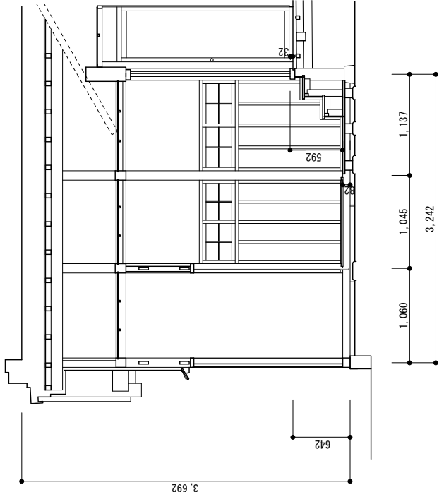
桁行断面図
