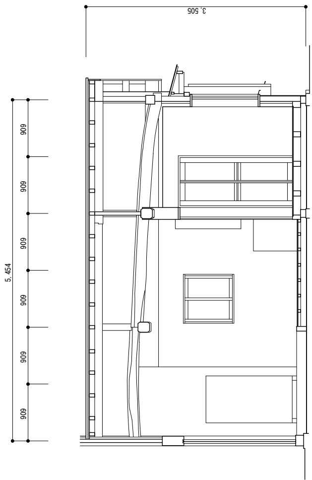
桁行断面図
