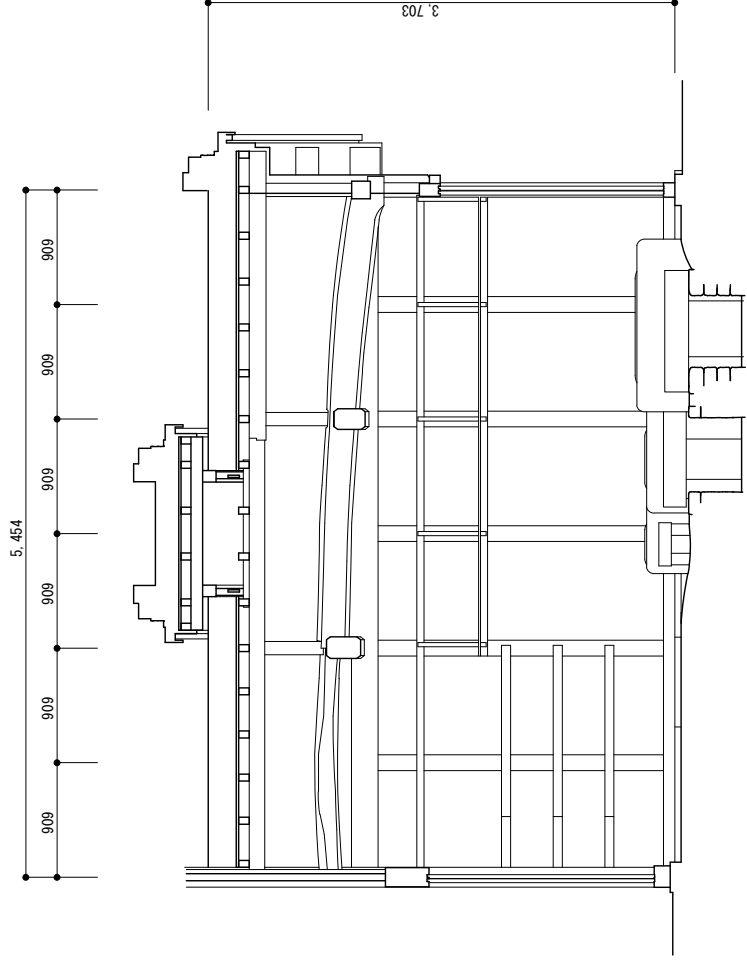
桁行断面図
