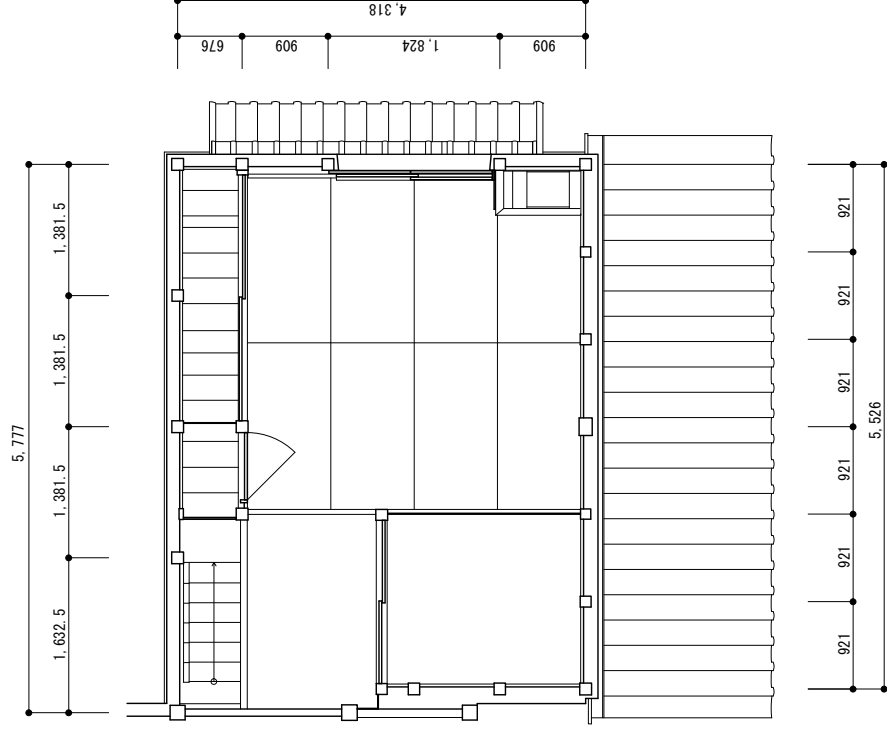
二階平面図
