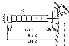
南塼西半 断面図
