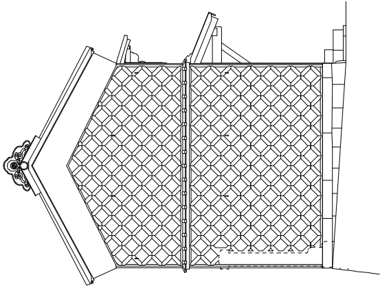
西立面図
