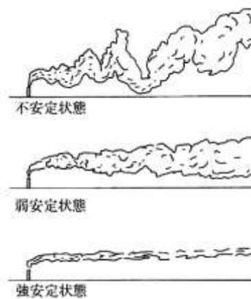
図 3.1.9 大気安定度の模式図
