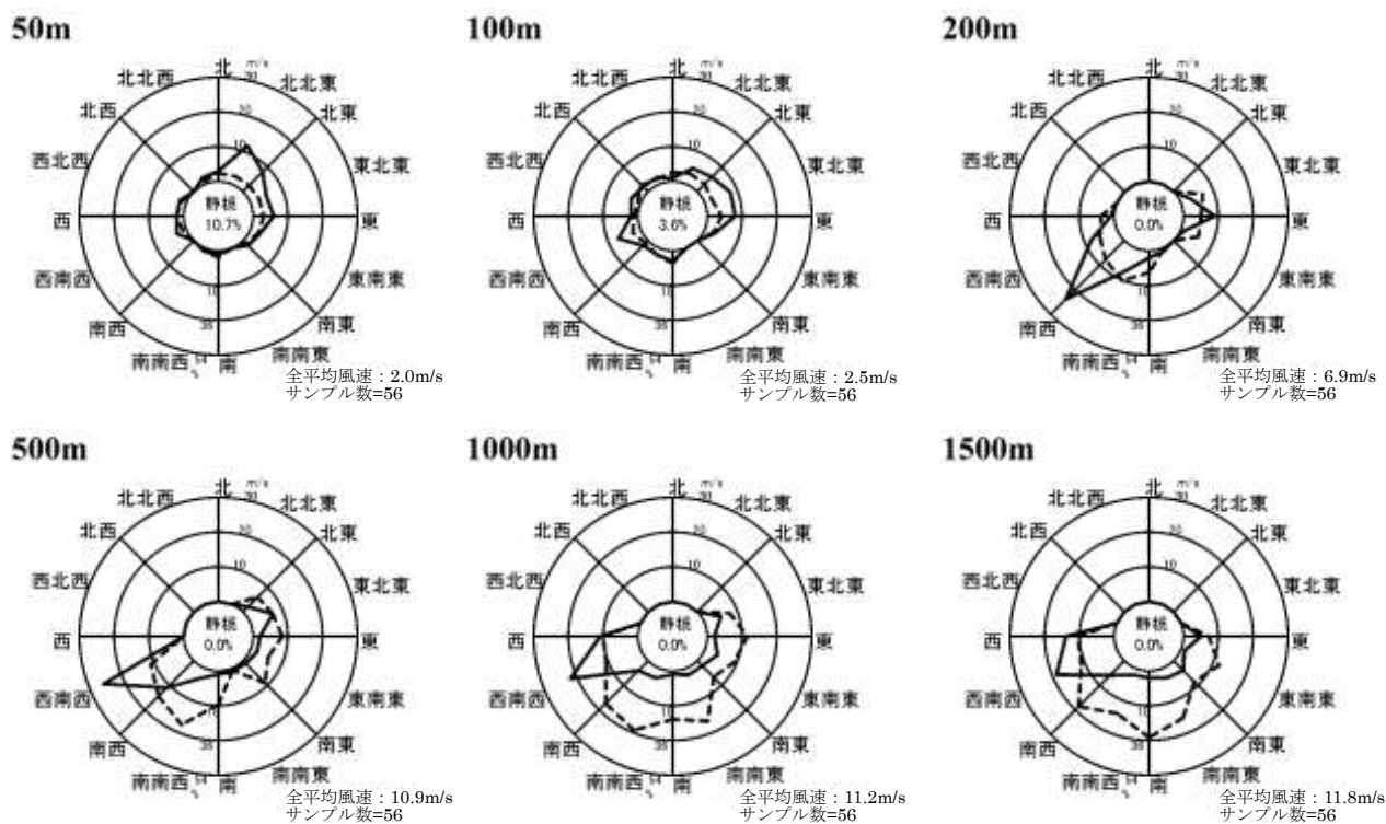
図 3.1.7 風向風速の鉛直分布 (夏季)
