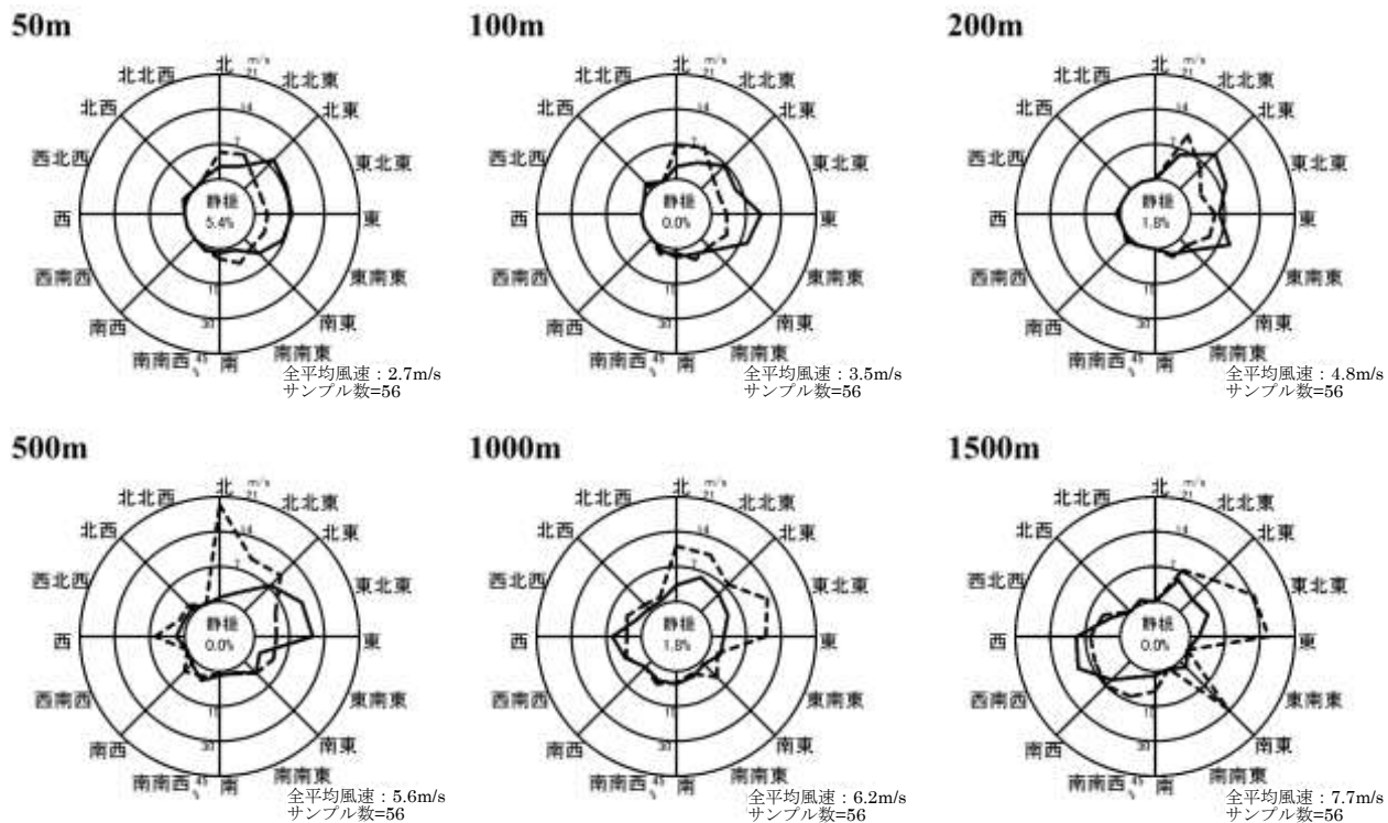
図 3.1.6 風向風速の鉛直分布 (冬季)
