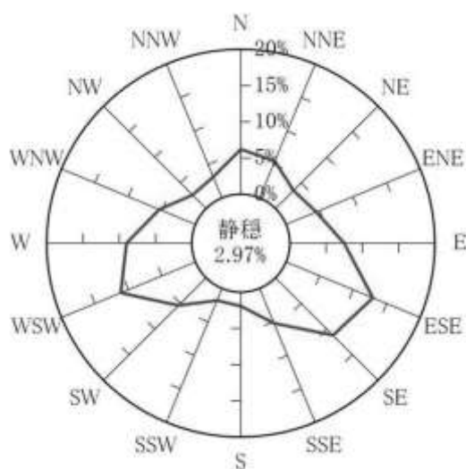
図 3.1.10 気象庁三島特別地域気象観測所の風配図（平成 26 年）
