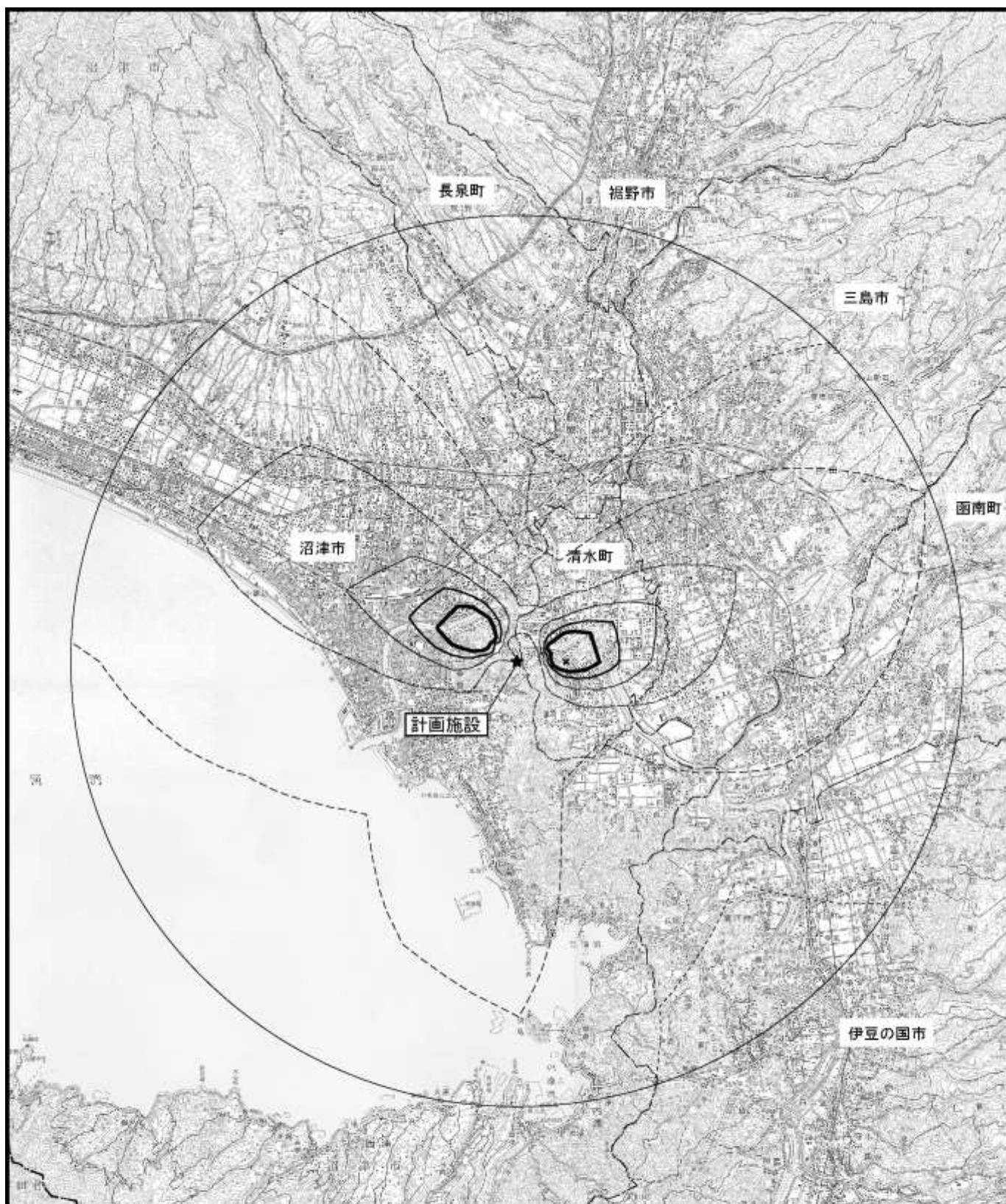
図3.1.13 大気質予測結果（窒素酸化物年平均寄与濃度）
