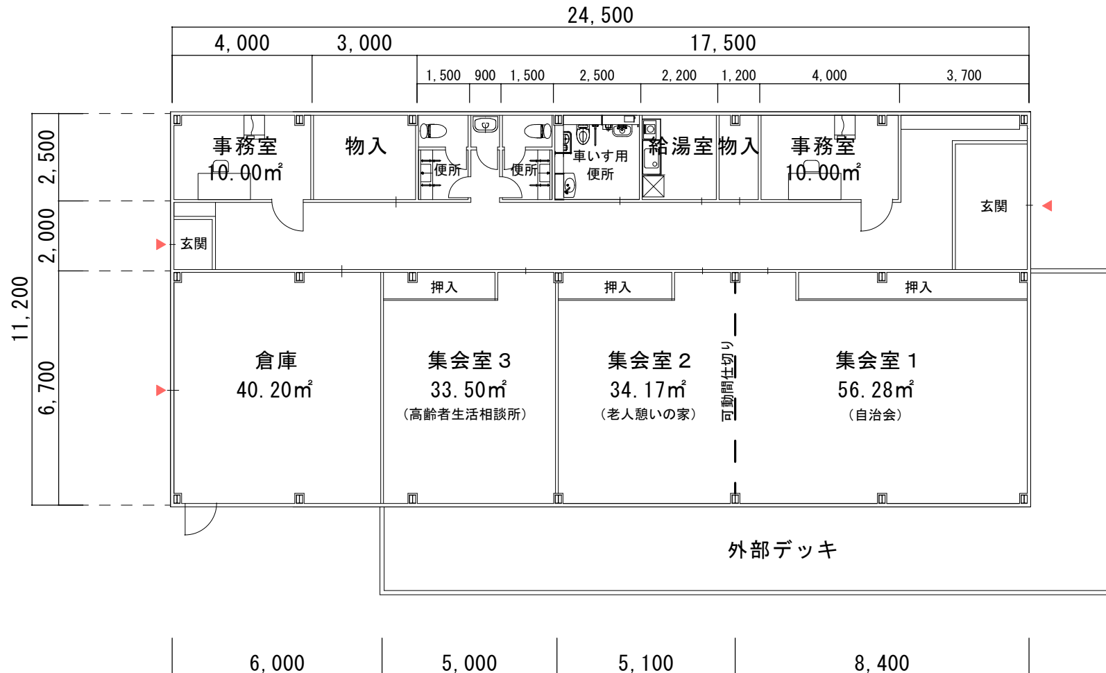
集会所の平面計画図案 1/150
