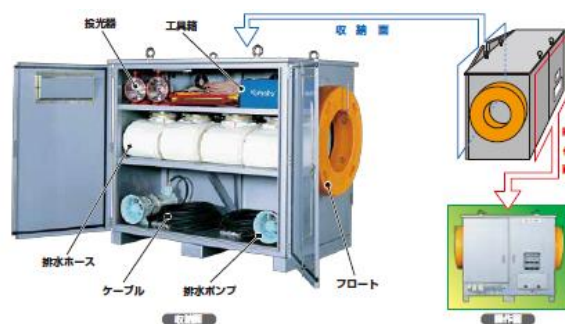
(排水ポンプパッケージイメージ)
